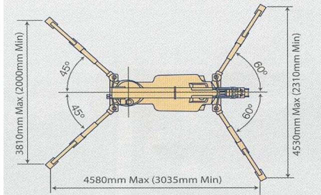
Le diagramme illustre les stabilisateurs en position maximum
